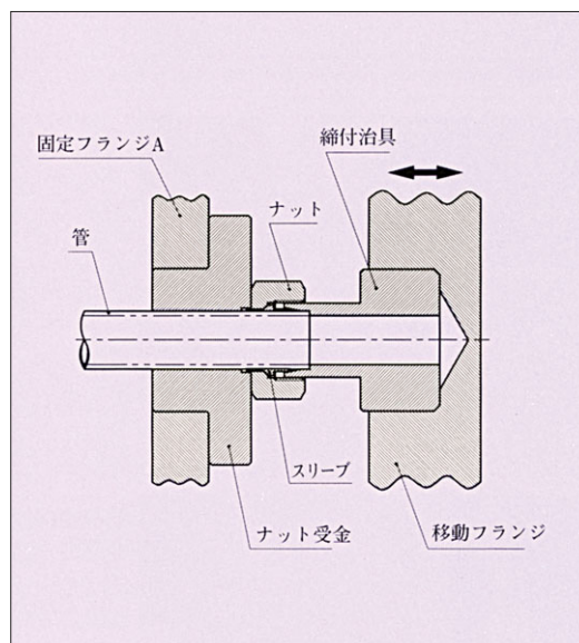
図-2 締付部詳細図
