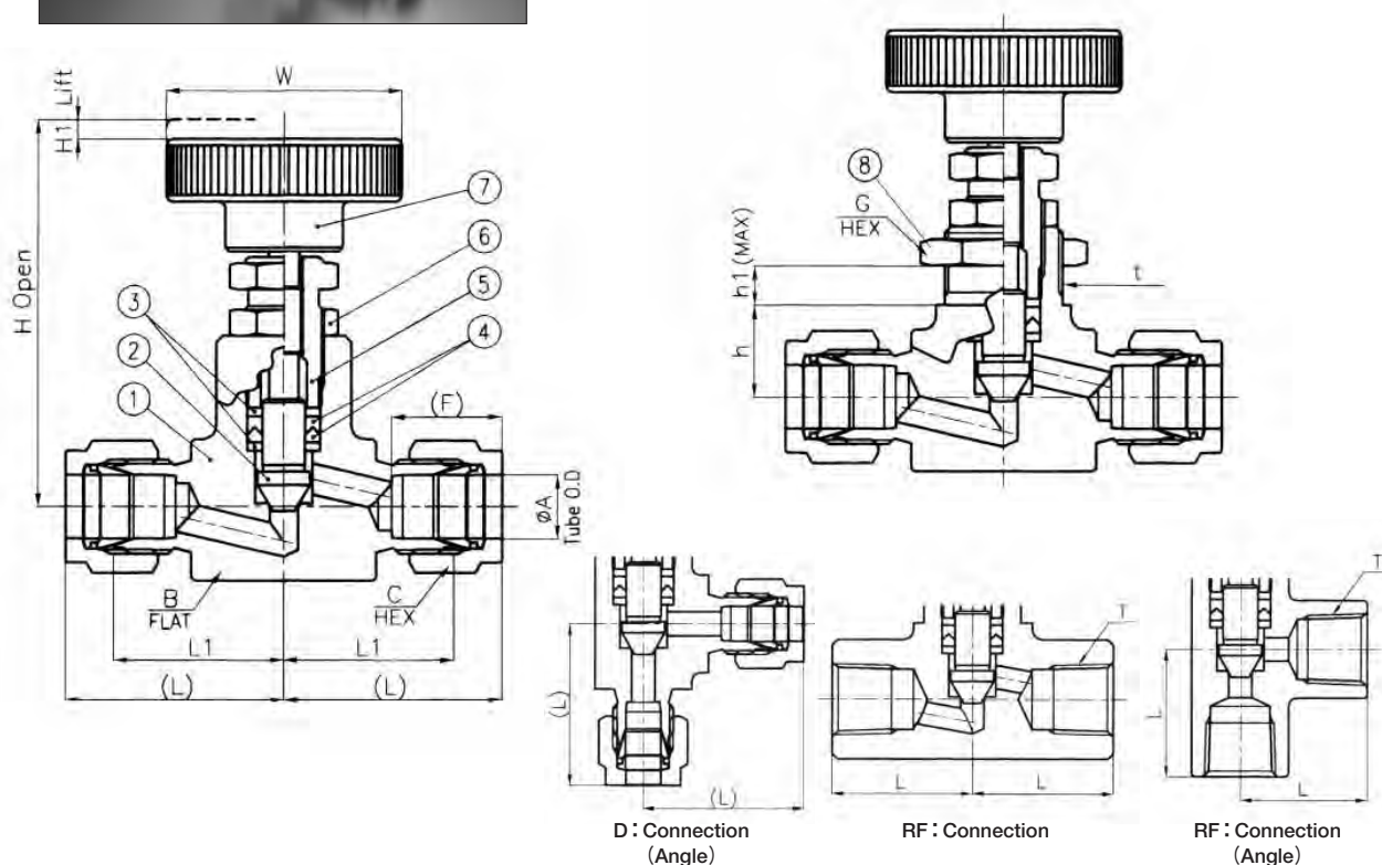
寸法表 BI-LOK 接続／Dimensions BI-LOK End
